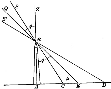
Fig. 7—The gnomon
